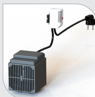
Chauffage (résistance thermostatée RCA)
